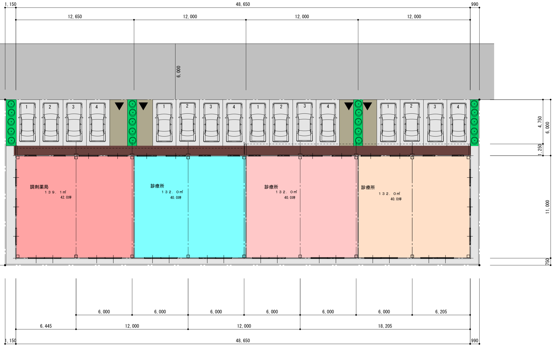
配置平面図
